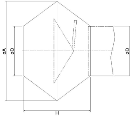
Detail Deflektorkopf
